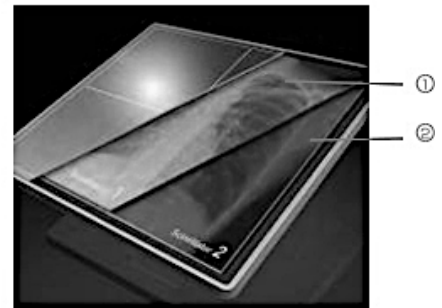
「CALNEO Dual」は、特性の異なる2種類のX線検出部（使用している蛍光体は、X線入射方向から①CsI、②GOSの順）を積層している。
